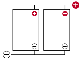
PARALLELSCHALTUNG:
